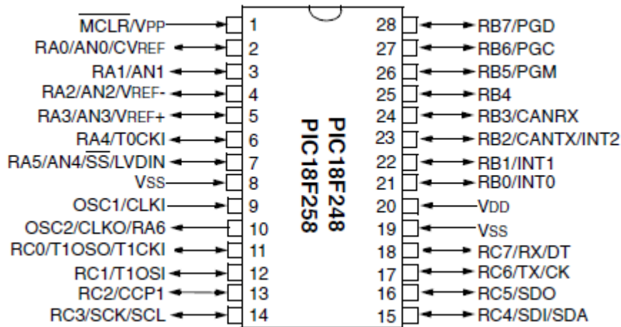
Ilustração 16. PIC18F258
