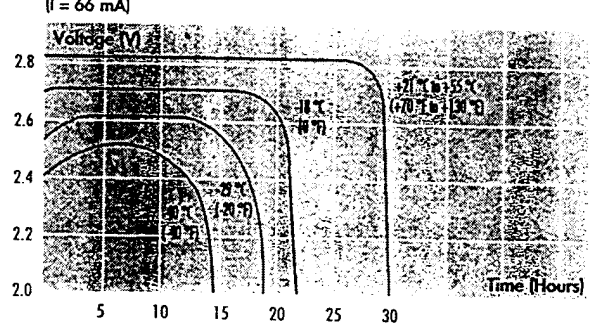
LO35 SX - Discharge profiles (I = 66 mA)
