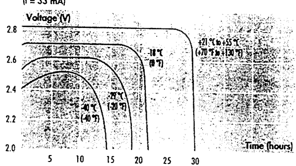
LO34 SX - Discharge profiles (I = 33 mA)
